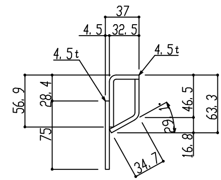
端上げ材詳細図
